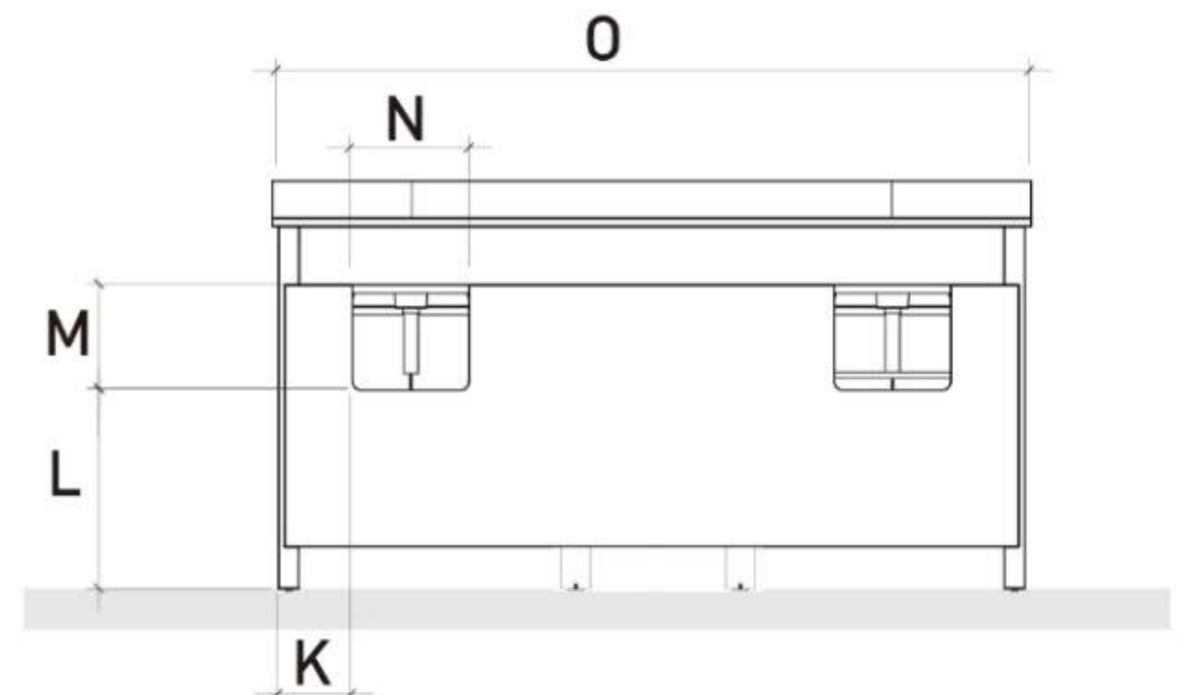
REAR VIEW VUE ARRIÈRE VISTA TRASERA
