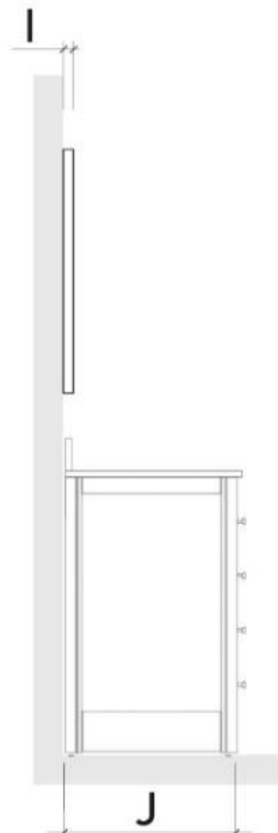
LEFT SIDE VIEW VUE GAUCHE VISTA IZQUIERDA
